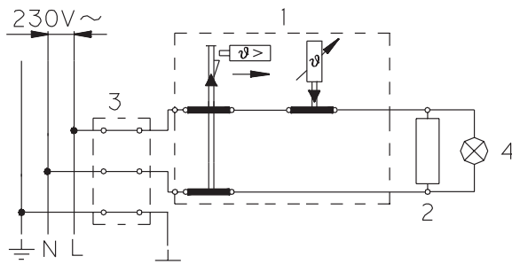
Схема електричного підключення
